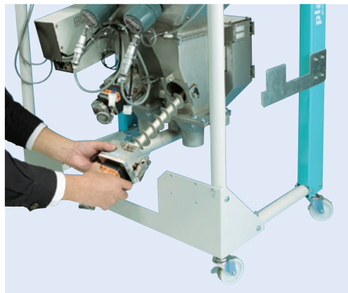
スクリュフィーダー部 Screw Feeder
